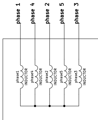
moteur pap à 5 phases
